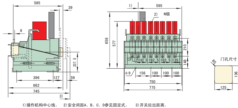
图16-8 DW17D-2900/4 (In=2900) 四极抽屉式接线
