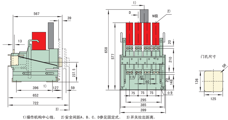
图16-7 DW17D-2900/4 (In=2000、2500) 四极抽屉式接线
