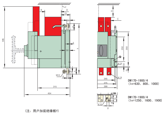
图16-2 DW17D-1900/4 (In=630~1900) 四极固定式垂直接线
