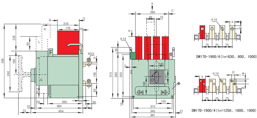
图16-1 DW17D-1900/4 (In=630~1900) 四极固定式水平接线
