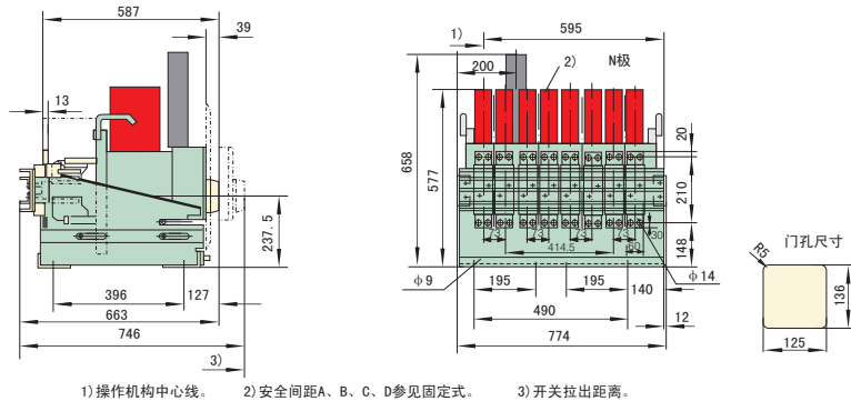
图16-8 DW17D-2900/4 (In=2900) 四极抽屉式接线
